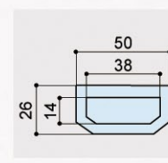
Dimensions
